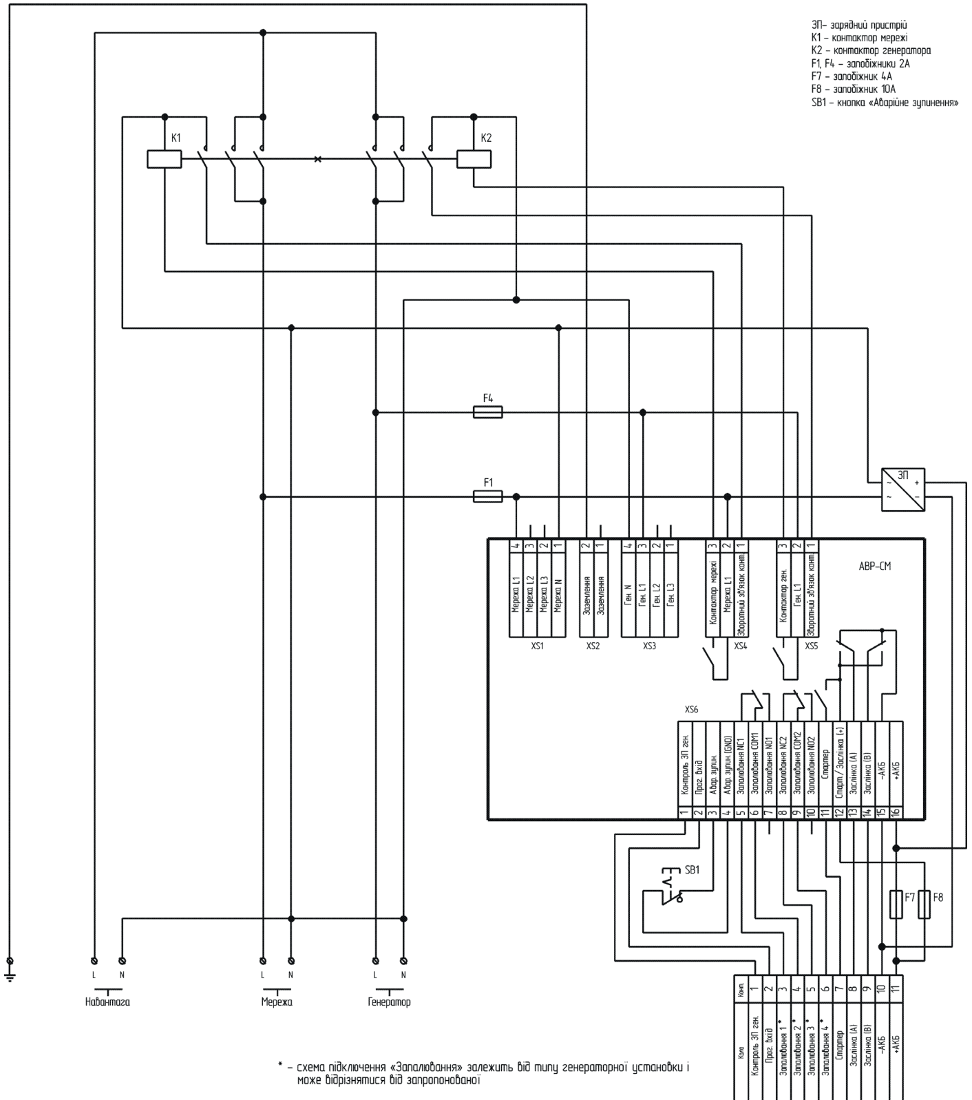
Рис. 6.4 – Схема підключення контролера для конфігурації AVR11 зі спільним нейтральним проводом
