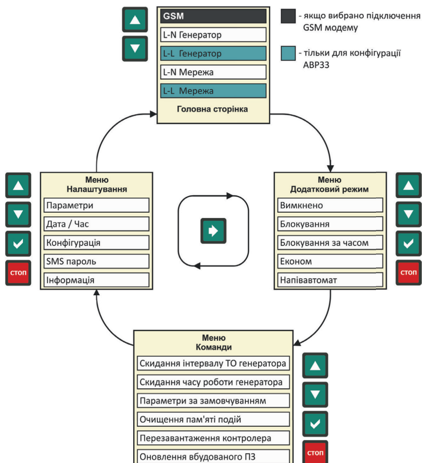
Рис. 5.3 – Структура індикації на дисплеї
