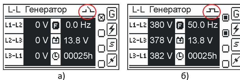
Рис. 5.8 – Індикація стану програмованого входу: а) розімкнутий; б) замкнутий
