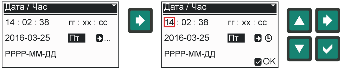
Рис. 5.16 – Меню «Дата/Час»
