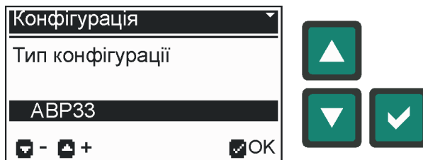
Рис. 5.18 – Меню «Конфігурація»
